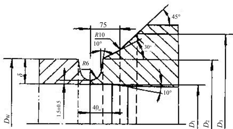
图 E.3 U(1)形坡口型式
